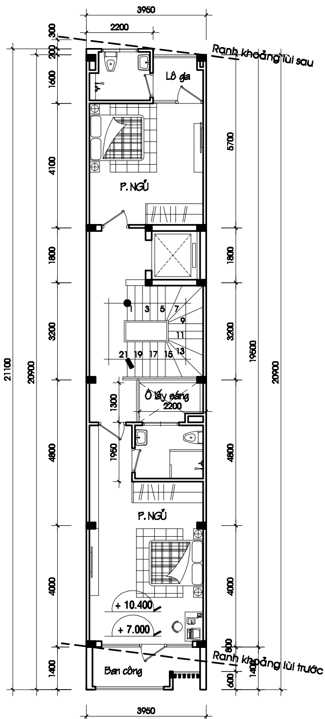
● MẶT BẰNG TẦNG 2, 3 TL : 1/ 100
