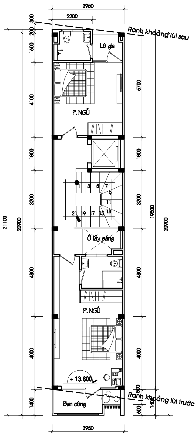
● MẶT BẰNG TẦNG 4 TL : 1/ 100
